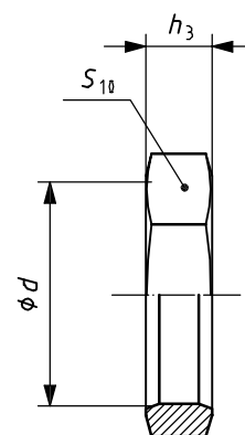
f) Bulkhead locknut (BHLN)
